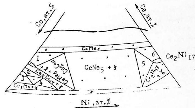
Рис.2. Схема расположения фазовых областей в системе Ce---Ni---Co---Mo
